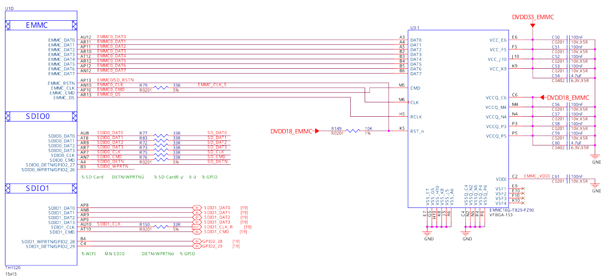
Fig. 3.28: 16GB eMMC
