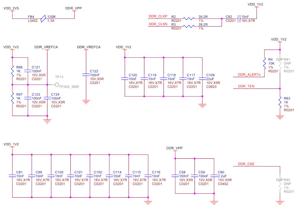
Fig. 3.40: DDR power
