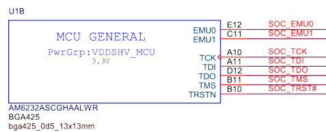
Fig. 3.43: JTAG
