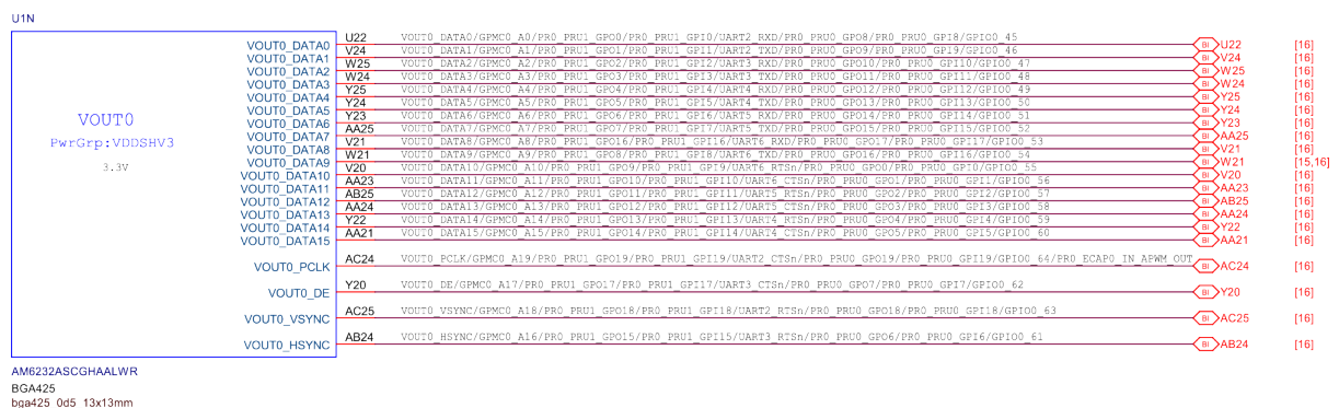
Fig. 3.18: GPIO VOUT0
